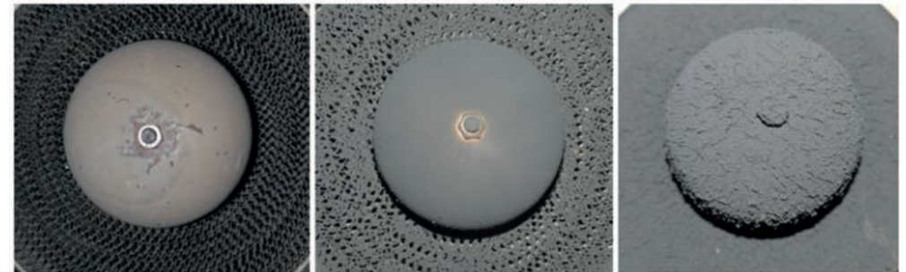
Abbildung 6: Sauberer Katalysatorinsatz (Abbildung links), zu reinigender Katalysatorinsatz mit bereits reduzierter Funktion (Abbildung Mitte), sehr stark beladener Katalysatorinsatz, nicht mehr funktionsfähig (Abbildung rechts)
